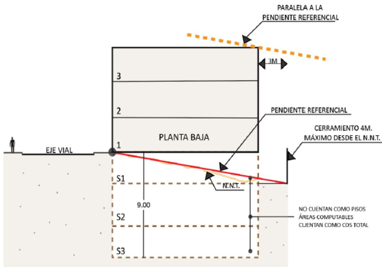
Ilustración 6: En línea de fábrica con pendiente negativa
