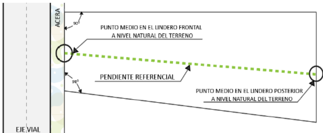
Ilustración 2: Pendiente referencial en terrenos irregulares
