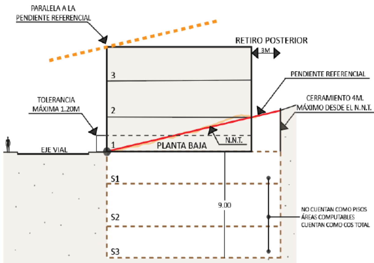
Ilustración 5: En línea de fábrica con pendiente positiva
