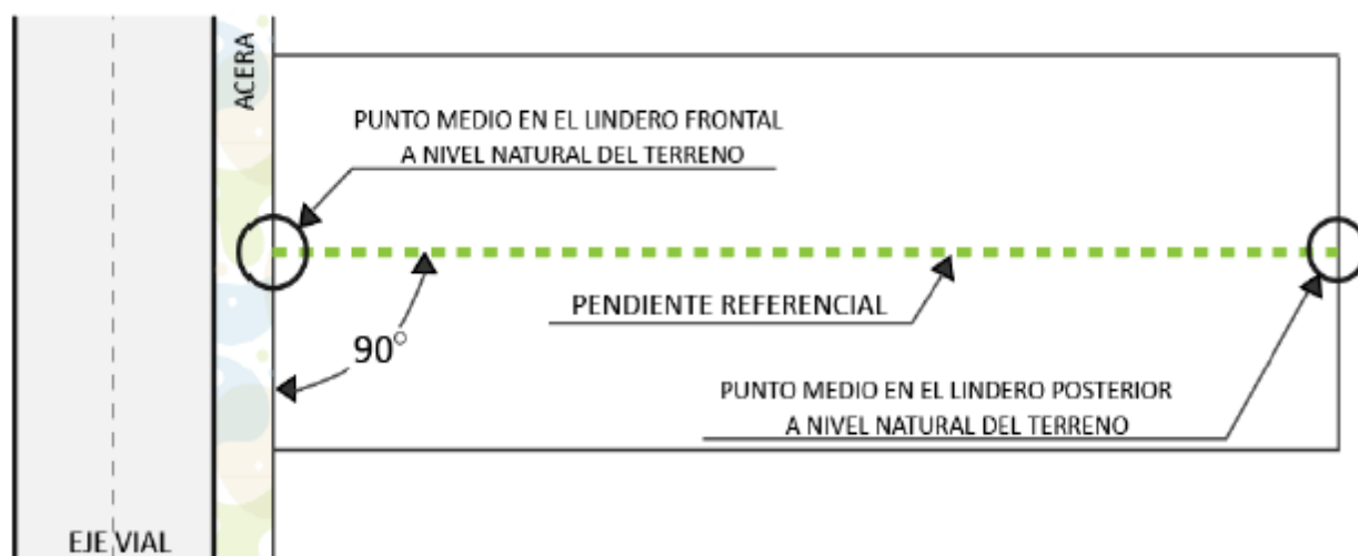
Ilustración 1: Pendiente referencial en terrenos regulares
