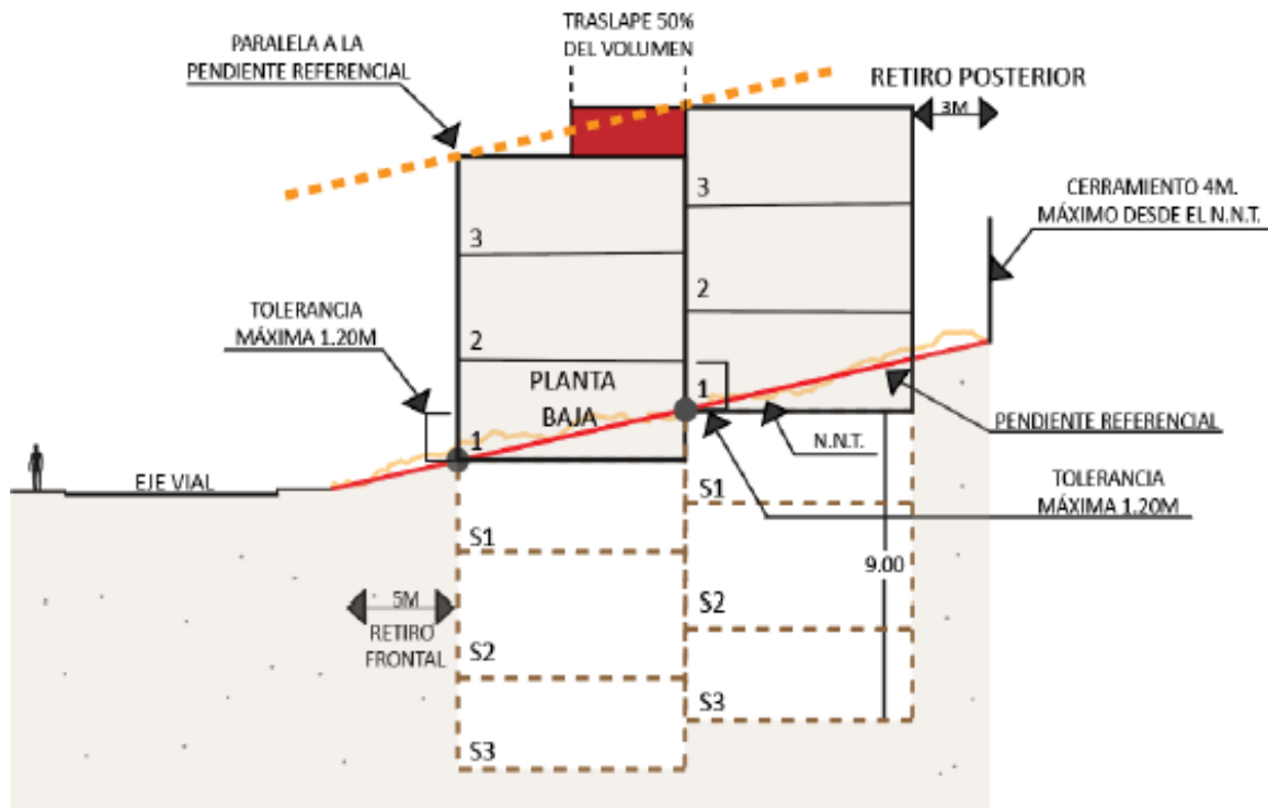
Ilustración 7: Con retiro frontal y pendiente positiva
