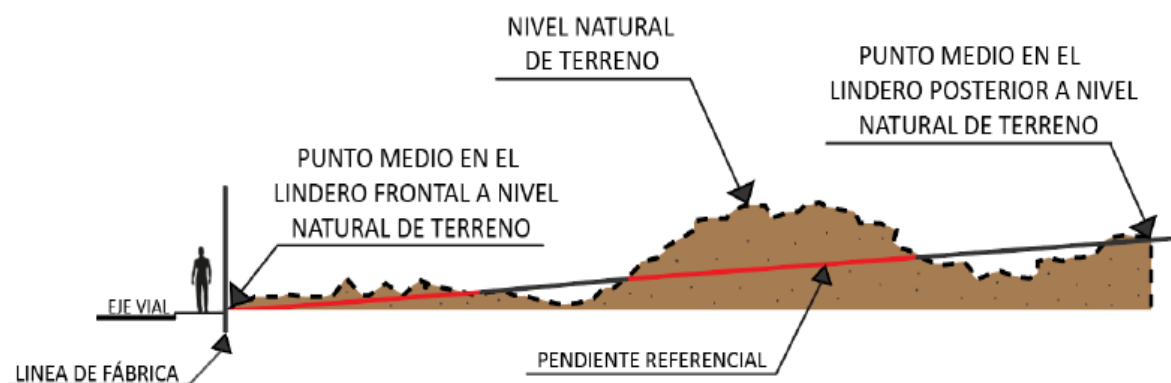
Ilustración 3: Corte de pendiente referencial
