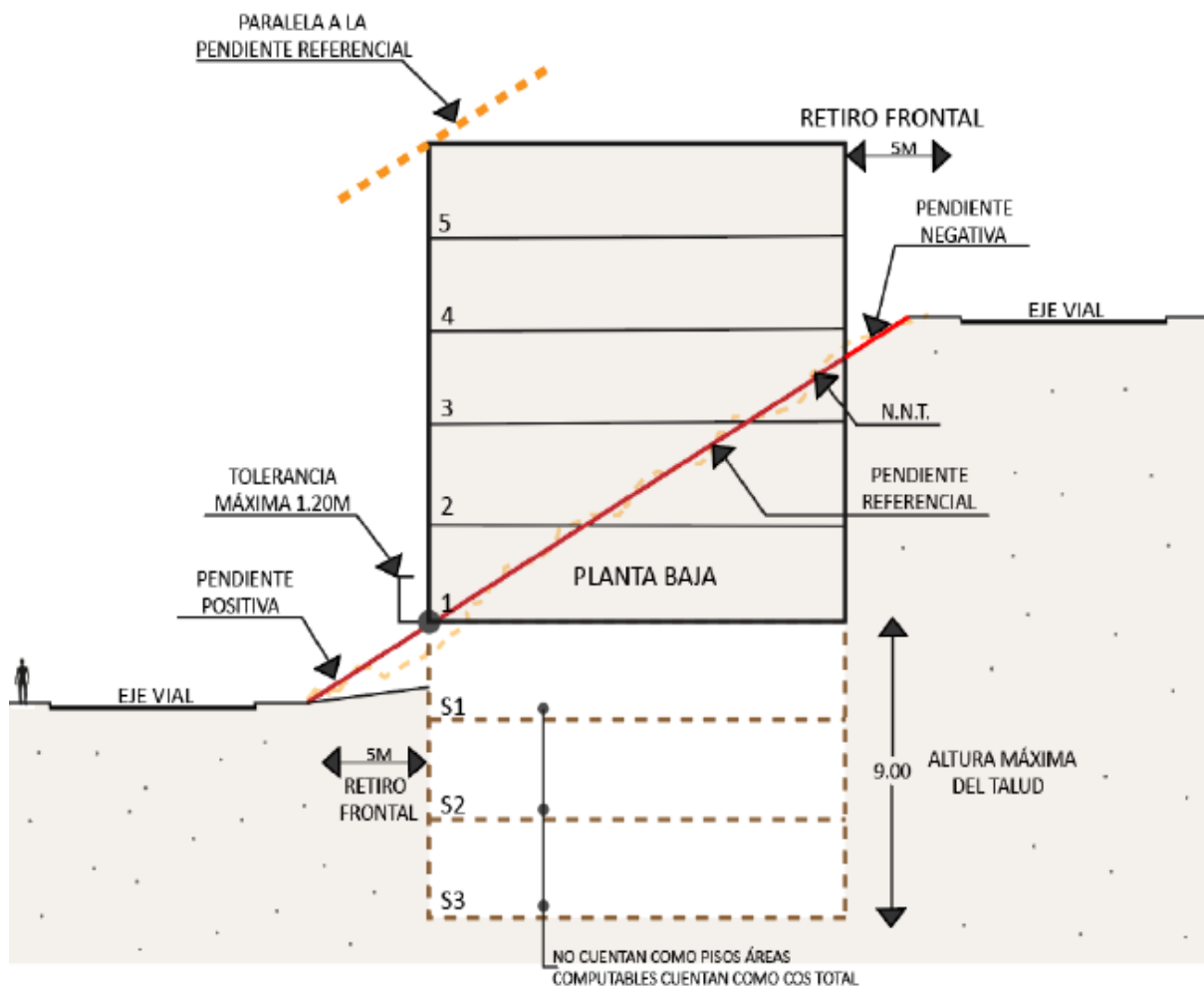
Ilustración 4: Edificaciones con pendiente positiva o negativa con retiro frontal hacia 2 vías.
